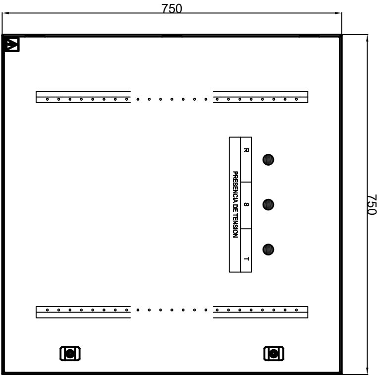
VISTA FRONTAL CON PUERTA
